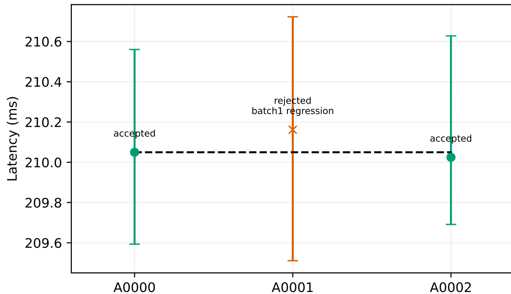
prefill
