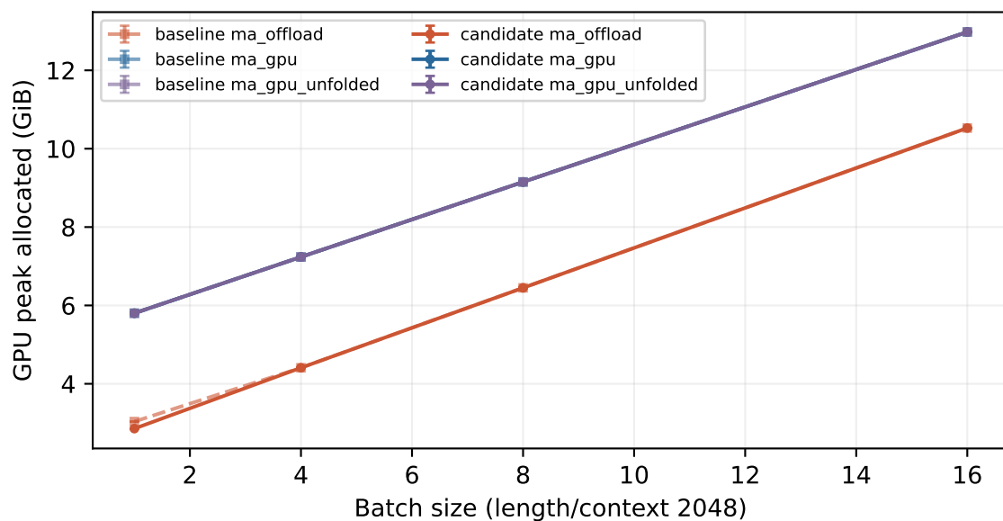
Prefill
