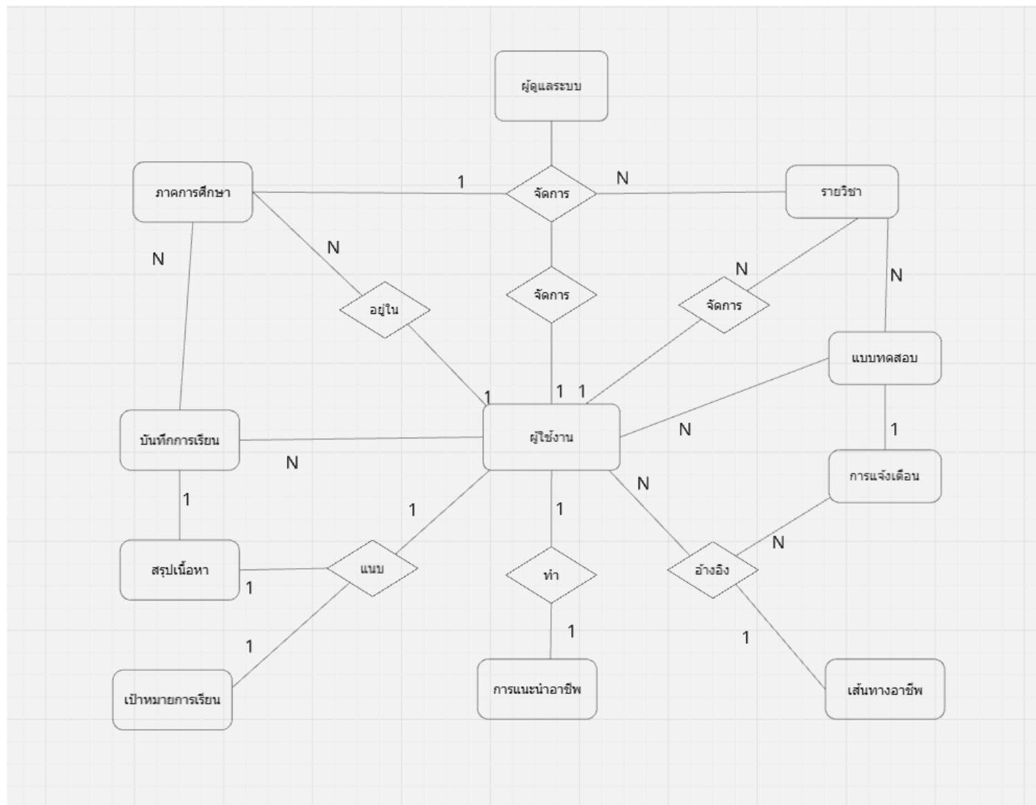
ER – Diagram
