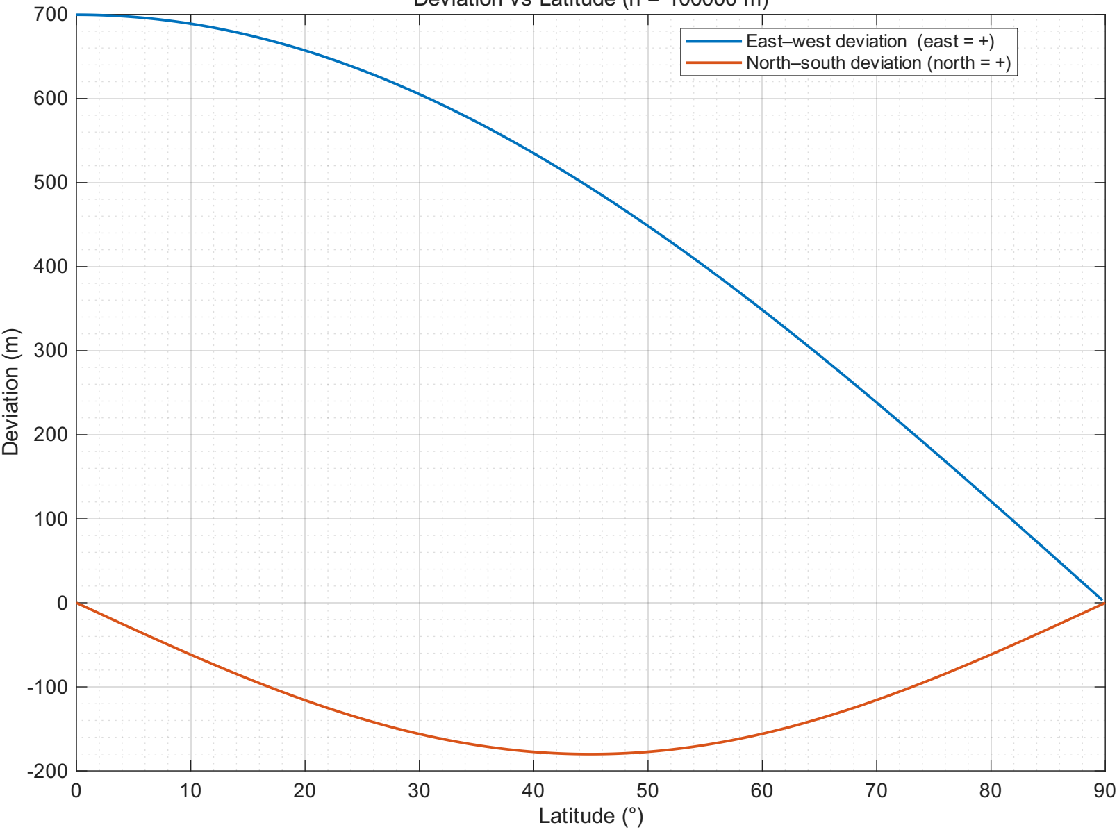
Deviation vs Latitude ( h = 100000 m)
