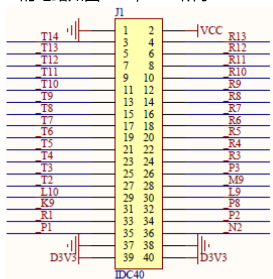
图 17.1 J1 扩展口原理图
