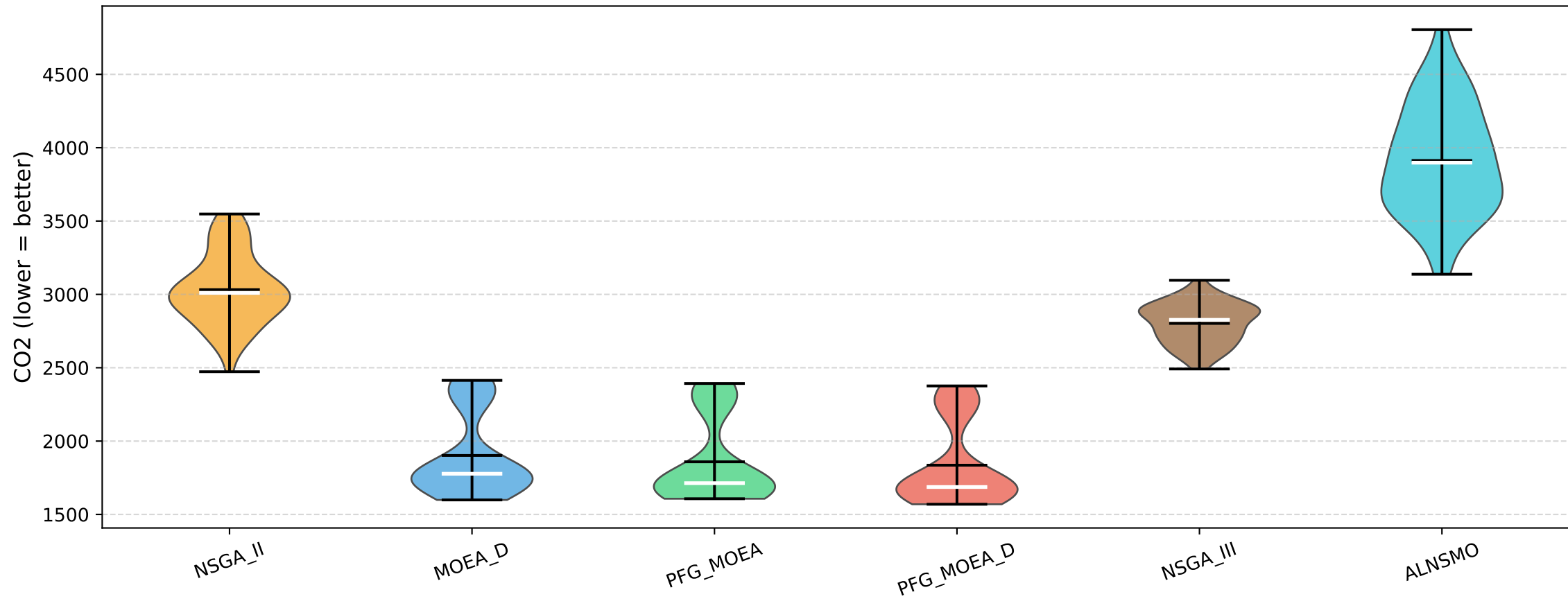
CO2 Distribution
