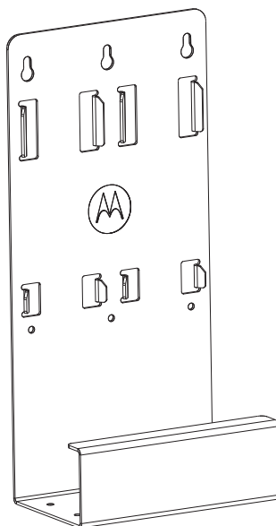
Figure 2 : Présentation du support de fixation (numéro de pièce : BR000628A01)
