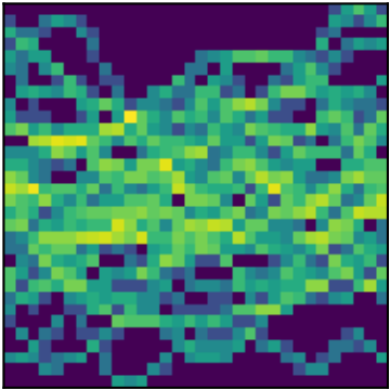
peak 7 P=2.1170d (LS)
