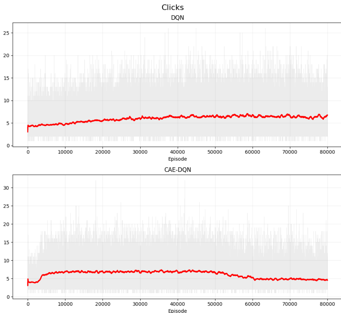
Gambar 4.2. Number of clicks dari pelatihan DQN dan CAE-DQN selama 80,000 episode
