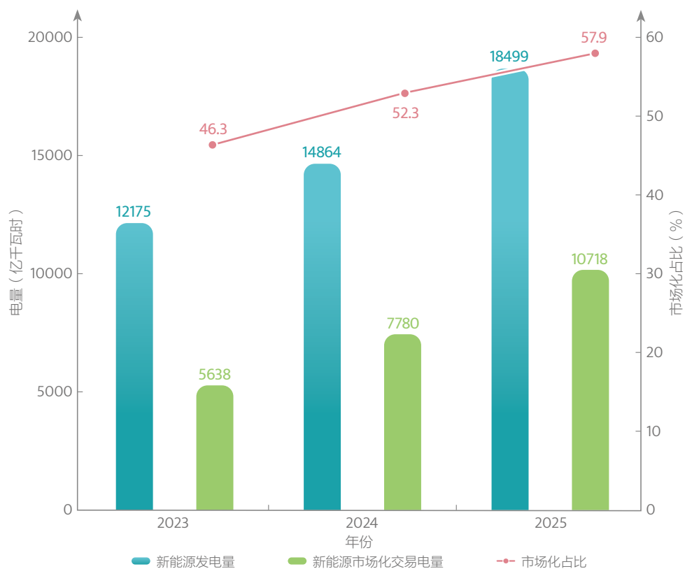
2023—2025年新能源市场化交易情况
