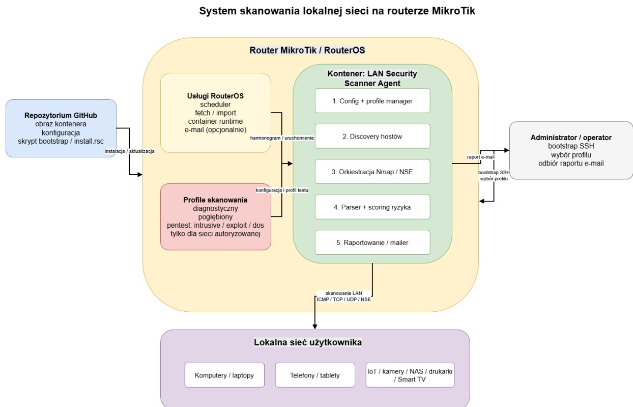
Rysunek 1: Architektura logiczna projektowanego systemu.
