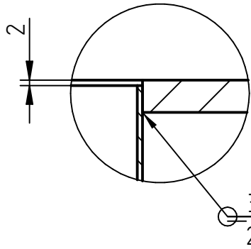
局部放大图 B 1:2
