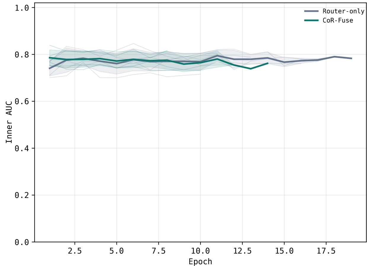
Inner-validation AUC
