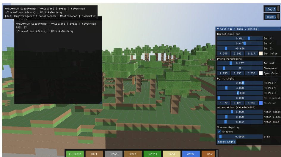
图 2: PCF 软阴影效果展示
