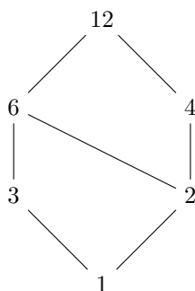
偏序集 (12 的正因数, 整除性)
