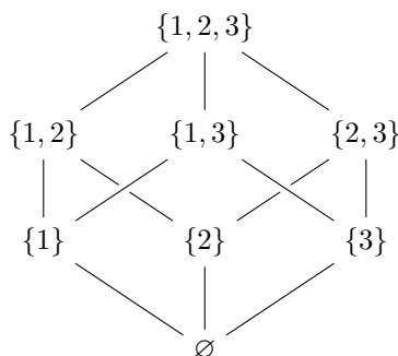
偏序集 (P(\{1, 2, 3\}), \subset)
