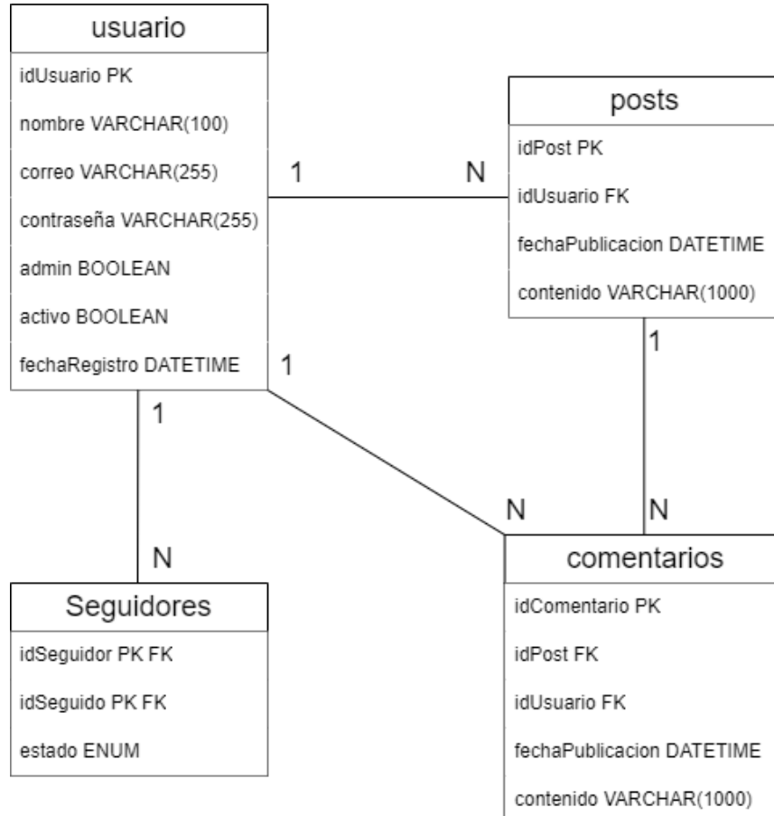
Esquema Relacional:
