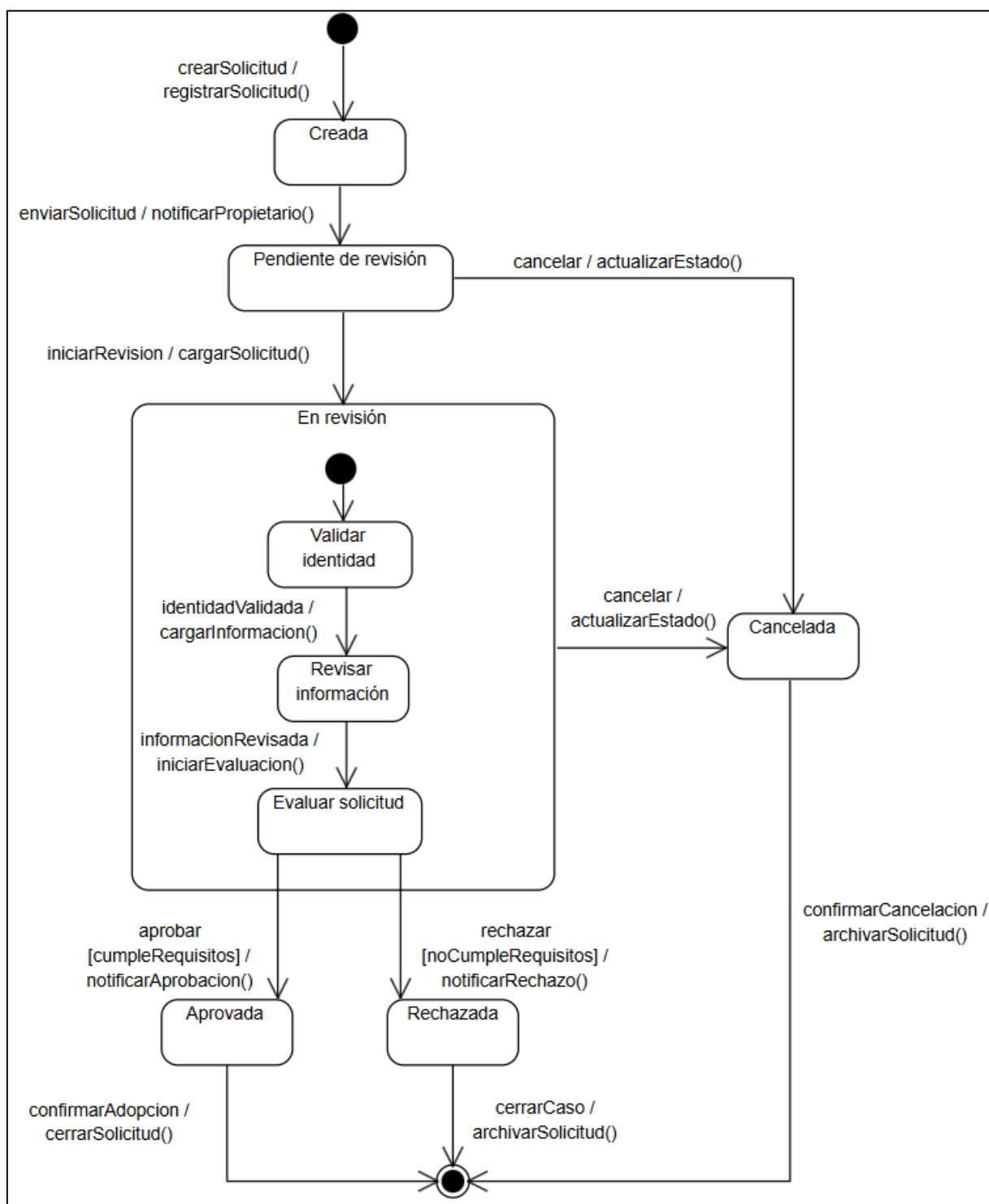
Figura 7: Diagrama de máquina de estados UML
