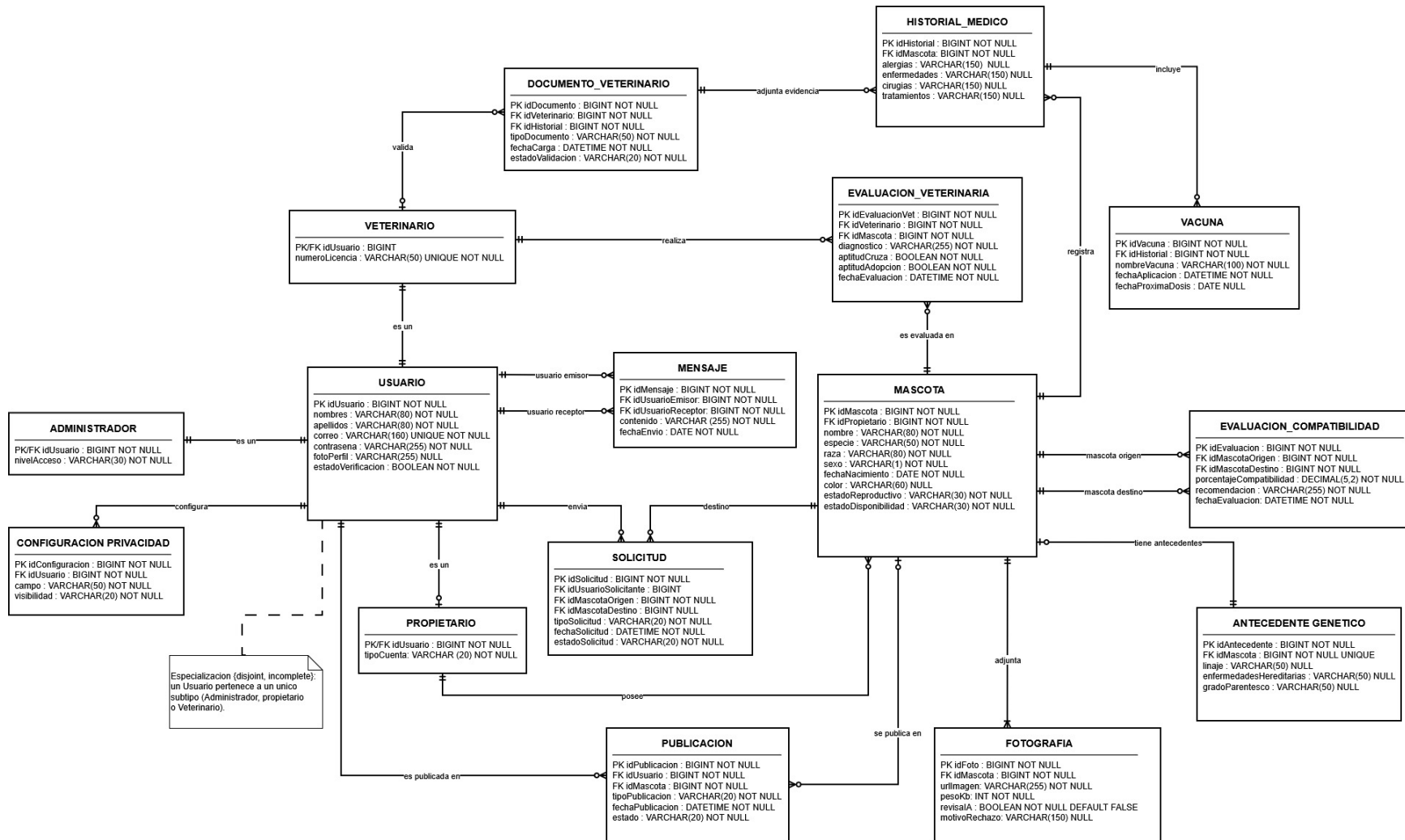
Figura 1: Diagrama Entidad-Relación
