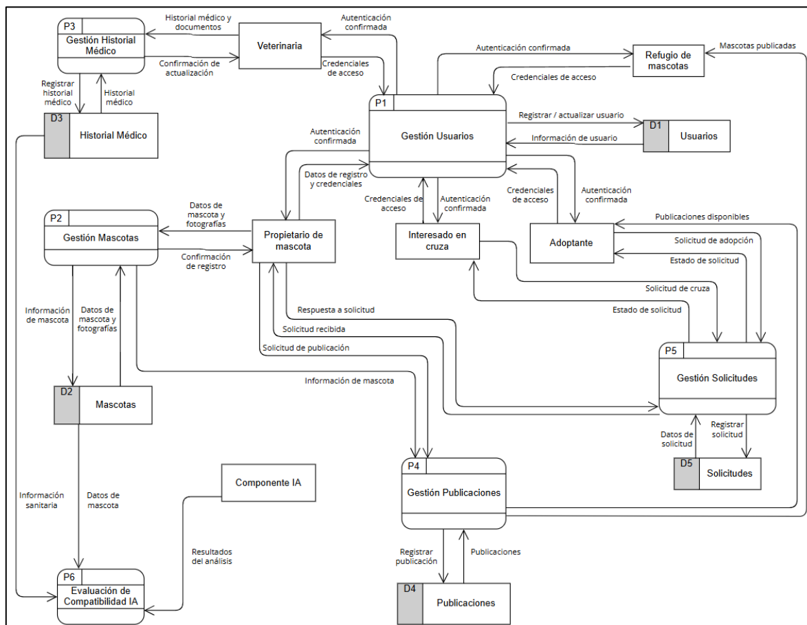
Figura 4: DFD Nivel 1
