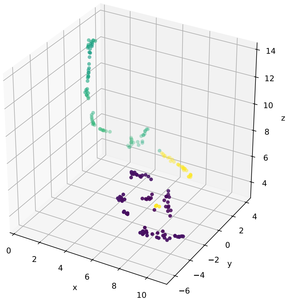
UMAP warm-start
