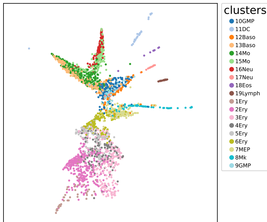
SMACOF init
