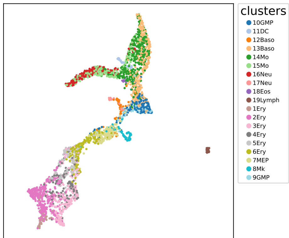
UMAP init
