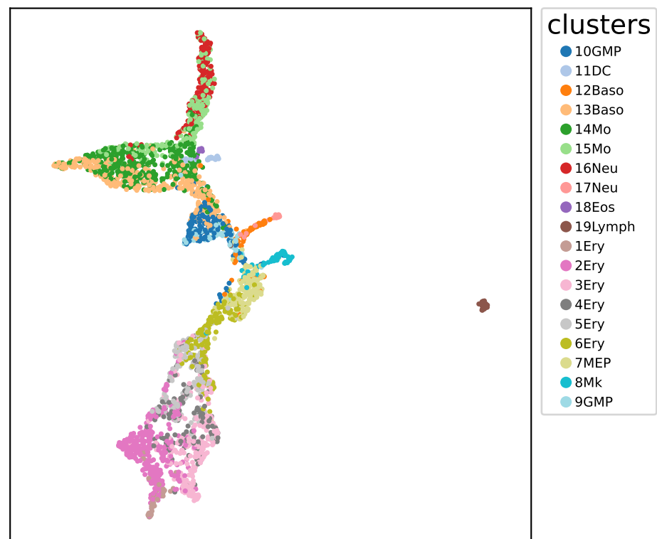
UMAP init
