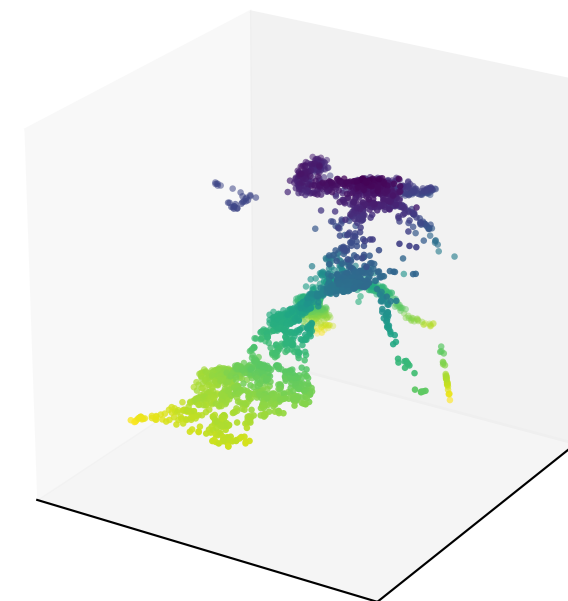
Path-frozen Randers alpha=0 (oblique)
