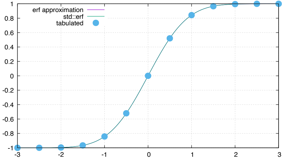
Error Function \text{erf}(x)
