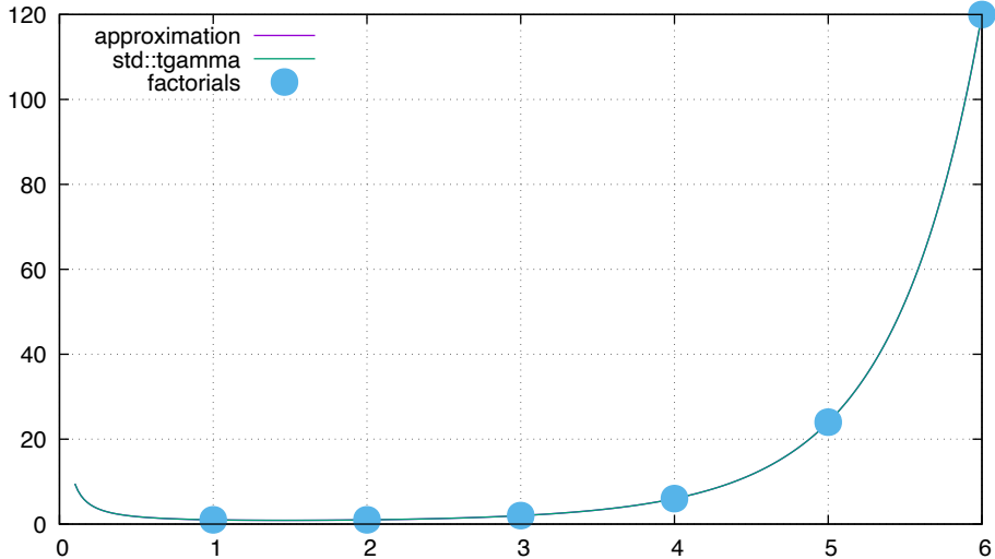
Gamma Function \Gamma(x)
