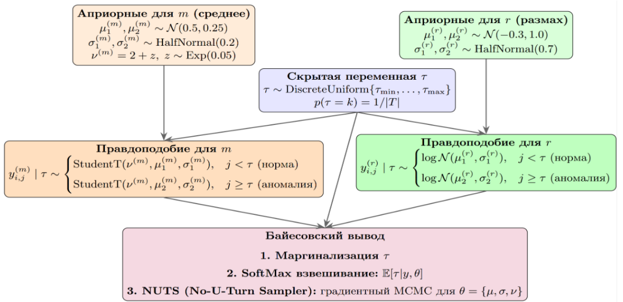
Рис. 6. Схема модели поиска точки разладки с priorными значениями параметров правдоподобия; в конкретном примере для среднего используется распределение Стюдента, а для размаха – логарифмически-нормальное.
