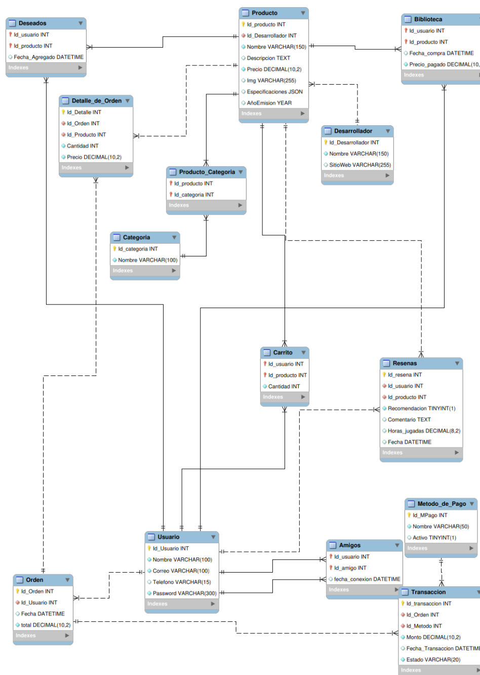
Figura 1. Modelo Entidad-Relación de la Plataforma
