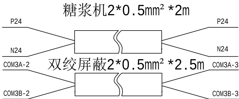
落杯落盖、糖浆机连接线缆图
