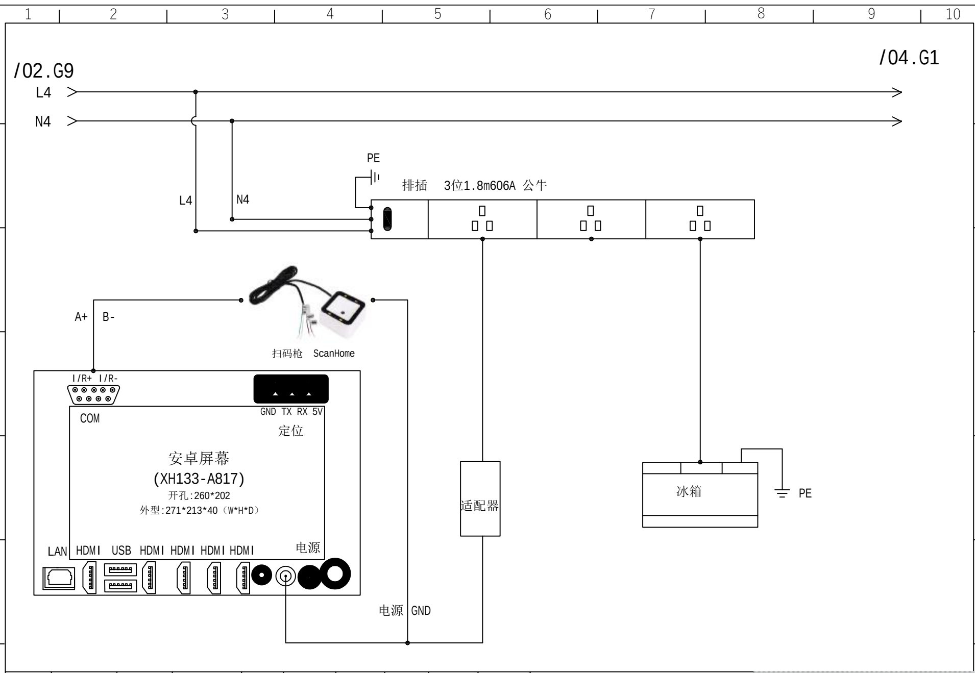
安卓屏幕及冰箱连接图
