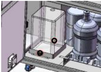
废液桶有桶检测感应传感器 3*0.5mm² *0m (P24、N24、X16)
