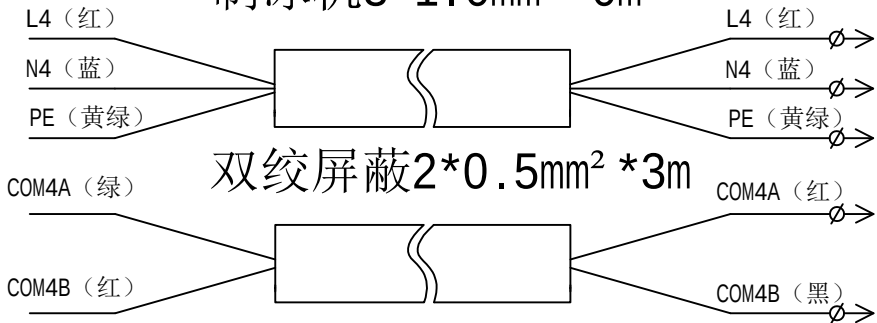
制冰机3*1.0mm 2 *0m
