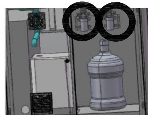
纯净水桶1液位低传感器 3*0.5mm² *0m (P24、N24、X14) 纯净水桶2液位低传感器 3*0.5mm² *0m (P24、N24、X18)
