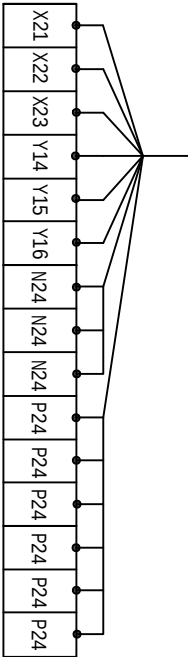
多芯电缆8*0.5mm²*2m
