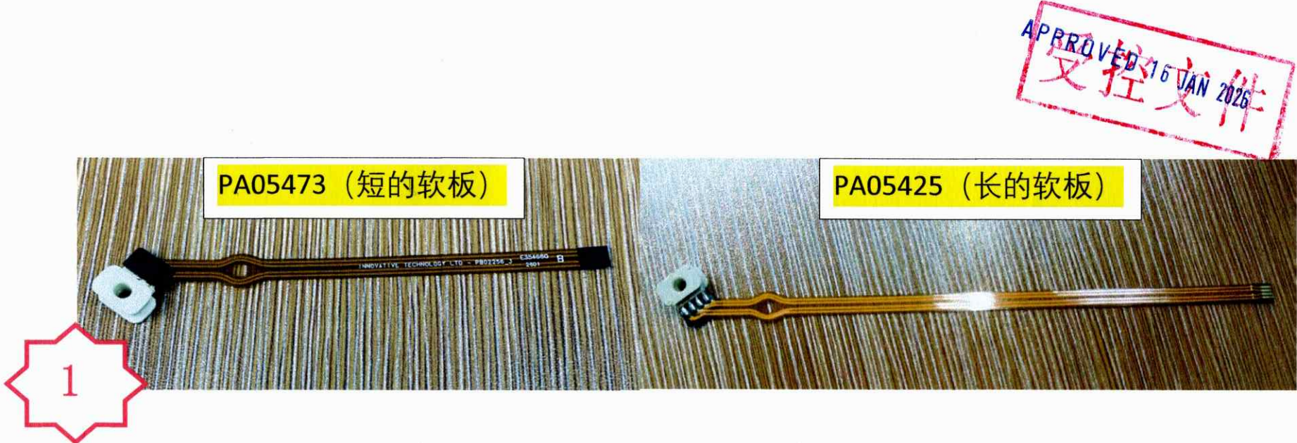
图一, PA05473/PA05425 组件识别
