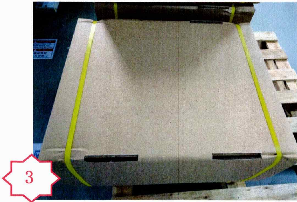
图三, 确认 PA05473/PA05425 无漏装后, 将 22 的内箱与外箱配合并打包装带待出货
