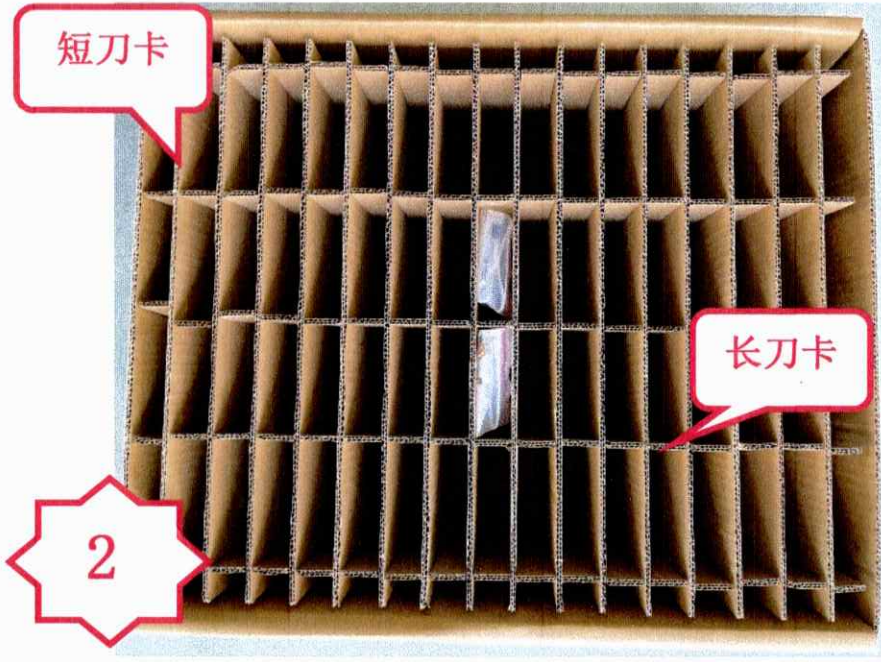
图二, 每 1 个气泡袋装 50 个组件, 每格放 1 袋 50 个, 每层 60 格 3000 个, 共 1 层, 同时在底层, 顶层各放 1 块隔板, 共 2 块。
