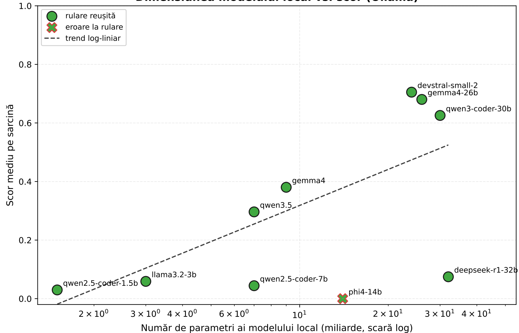
Dimensiunea modelului local vs. scor (Ollama)
