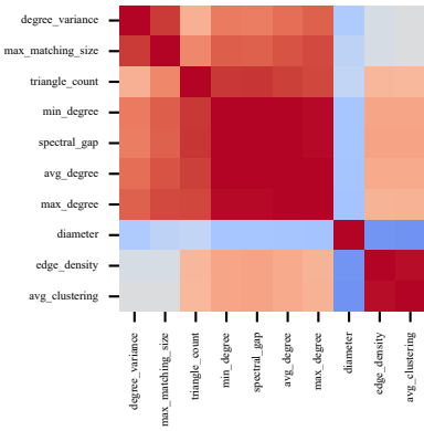
Erdős-Rényi
