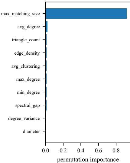
Erdős-Rényi
