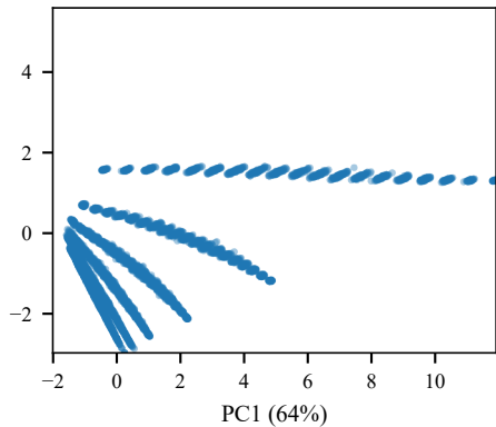
Erdős-Rényi
