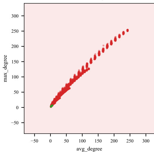
Erdős-Rényi
