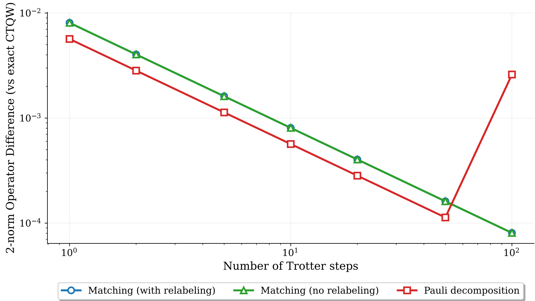
Sparse Non Bipartite Graph (5 qubits)
