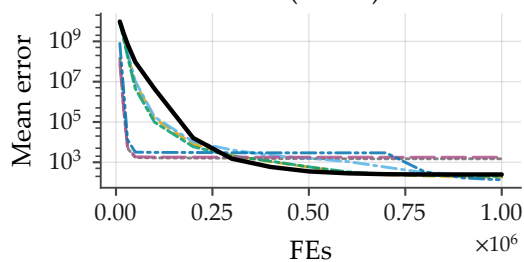
F19 (D=100)
