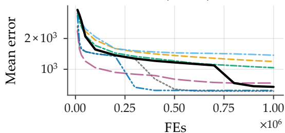
F23 (D=100)
