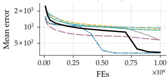
F21 (D=100)
