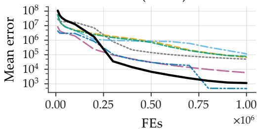
F18 (D=100)
