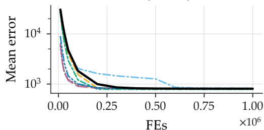
F25 (D=100)
