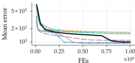
F24 (D=100)
