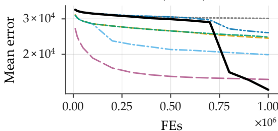
F22 (D=100)
