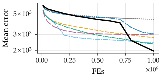
F20 (D=100)
