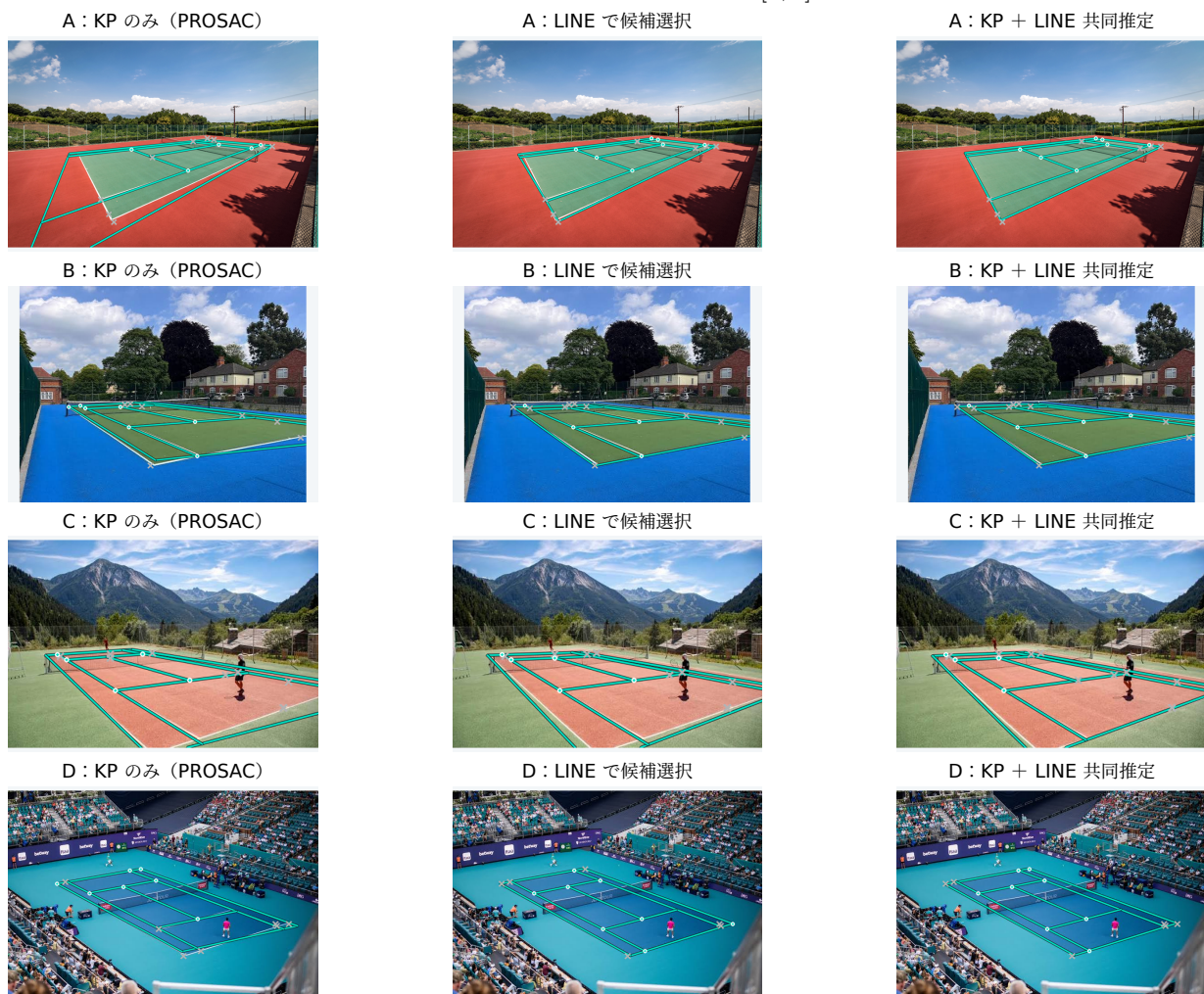
図 3 同一の保存推論を使う 3 段階の幾何復元。線は各段階の H、丸点は採用 KP、灰 × は不採用 KP である。最適化した候補のうち最良を選ぶため、中央の最良初期候補が必ず右の初期値とは限らない。定量的な予測間整合は表 2 に示す。
