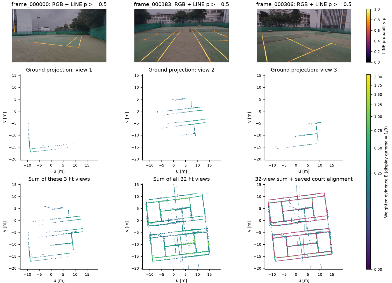
図2 各視点の LINE から投影・集約への過程。上段は校正済み実画像と実 LINE 確率の重畳、中段は同じ地面座標への各視点の投影。下段は表示 3 視点の和、全 32 当てはめ視点の和、保存コートとの重畳。16 保留視点は集約に含めない。地面図は白が支持なし、色域共通。細線を読むよう表示のみ 3 \times 3 セルの最大値へ縮約し、 \gamma = 1/3 とした。元の集約グリッドは保存値と完全一致した。当時の実画像入力・LINE 専用重み (epoch 19) の結果であり、未学習推論用の多タスク重み (epoch 17) とは区別する。
