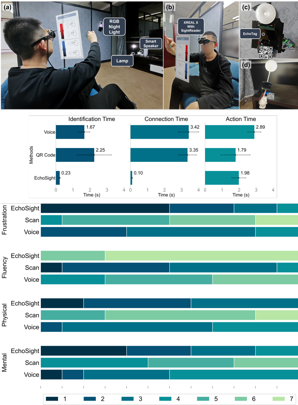
图 3.12 EchoSight 用户实验：实验场景、交互阶段、阶段耗时和主观问卷，拟组合原论文图 7至图 10
