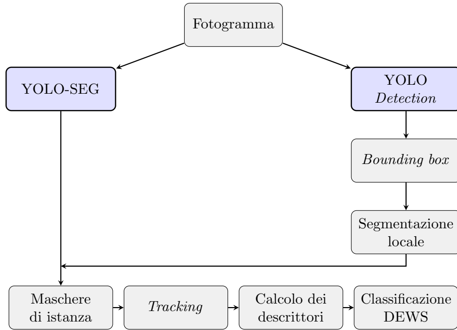
Figura 5.1: Percorsi di integrazione di YOLO-SEG e YOLO Detection nella pipeline DEWS
