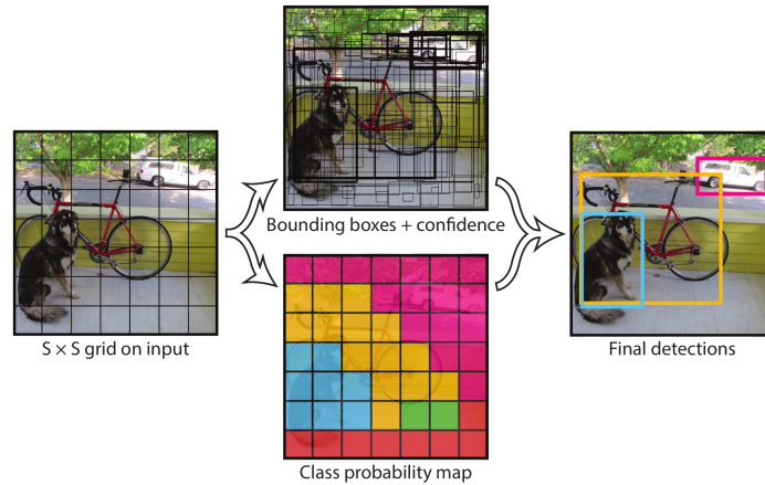
Figura 2.5: Rappresentazione delle predizioni di YOLOv1: griglia di ingresso, regioni con i relativi valori di confidenza, probabilità di classe e rilevazioni finali. Tratto da [14, Fig. 2]
