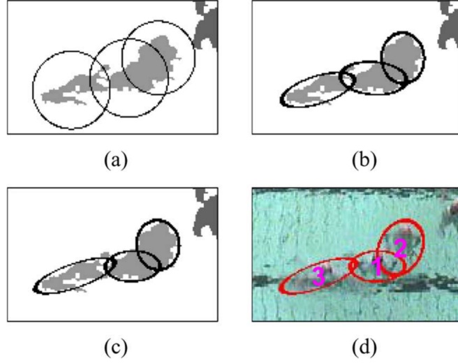
Figura 2.2: Processo di blob splitting adottato in DEWS: inizializzazione, adattamento delle ellissi e risultato finale. Tratto da [12, Fig. 8]
