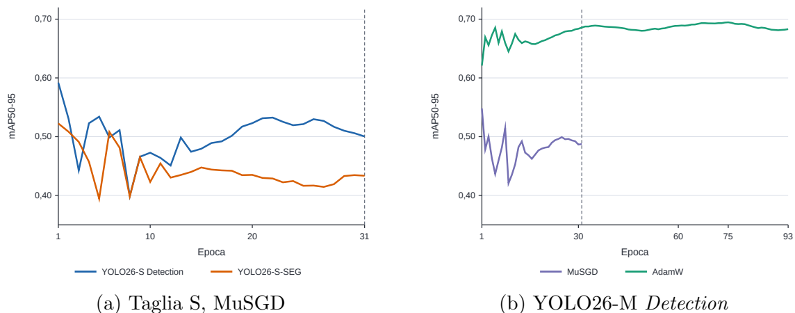
Figura 4.3: Andamento della mAP_{50:95} sul validation set durante gli addestramenti selezionati
