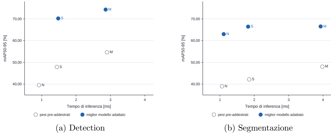
Figura 4.4: Rapporto fra mAP 50:95 e tempo di inferenza sul test set
