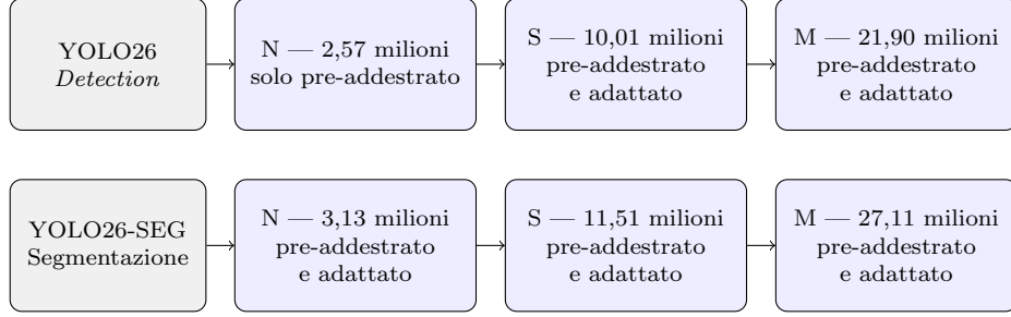
Figura 4.1: Varianti YOLO26 considerate e numero di parametri dei corrispondenti modelli pre-addestrati
