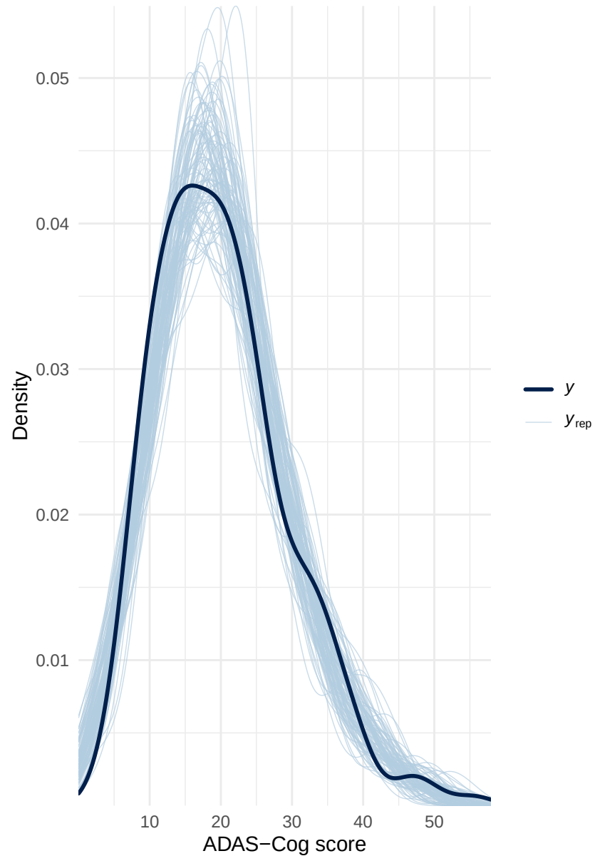
Posterior Predictive Check
