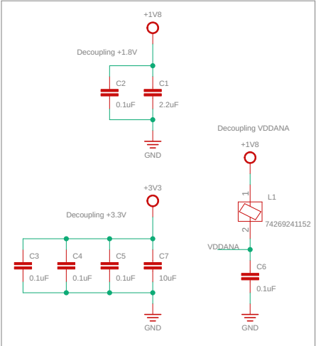
Decoupling
