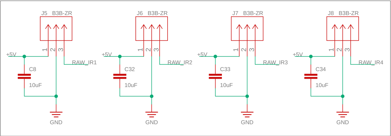
IR Sensors
