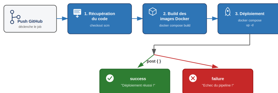
Figure 3 — Flux du pipeline Jenkins : les trois étapes s'exécutent séquentiellement, suivies du bloc post qui affiche un message de succès ou d'échec selon le résultat.
