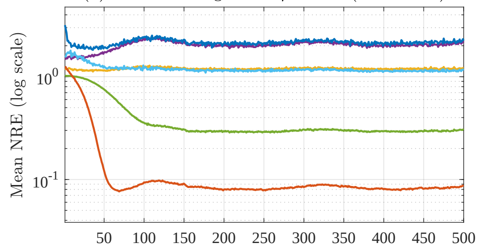
(d) Micro Convergence at \rho = 10\% (Rank = 10)
