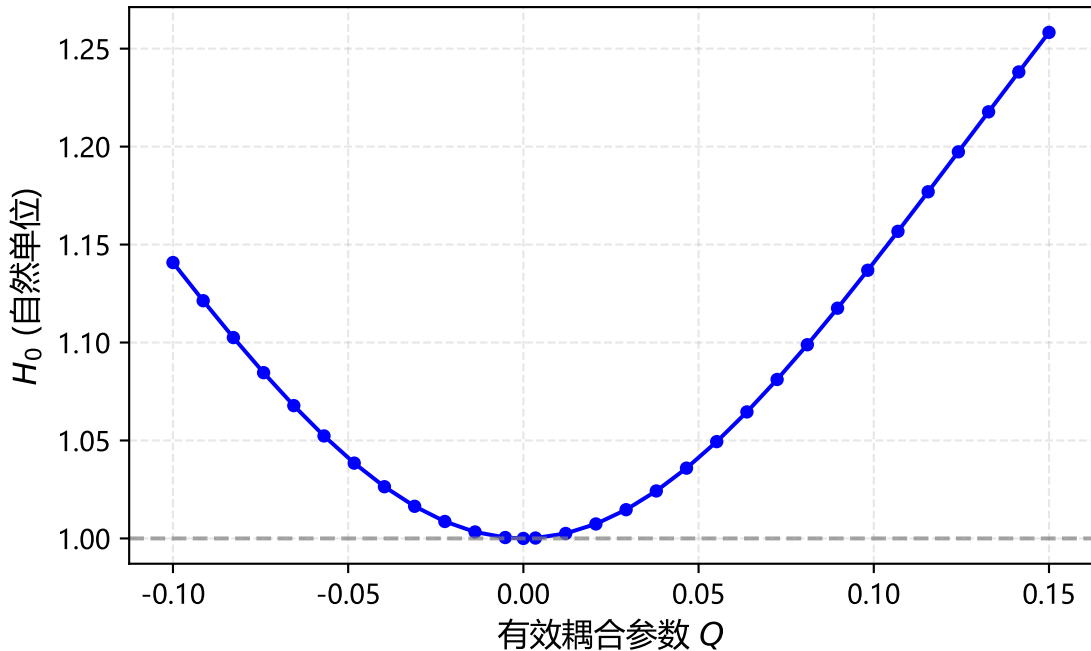
今天哈勃参数与耦合强度的关系
