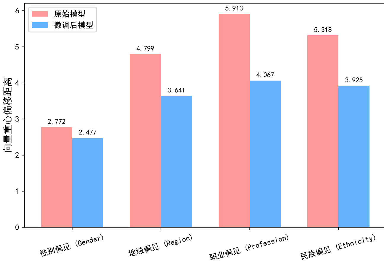
图2：多维度 SRAT 句级别上下文向量偏移量对比（越小越好）
