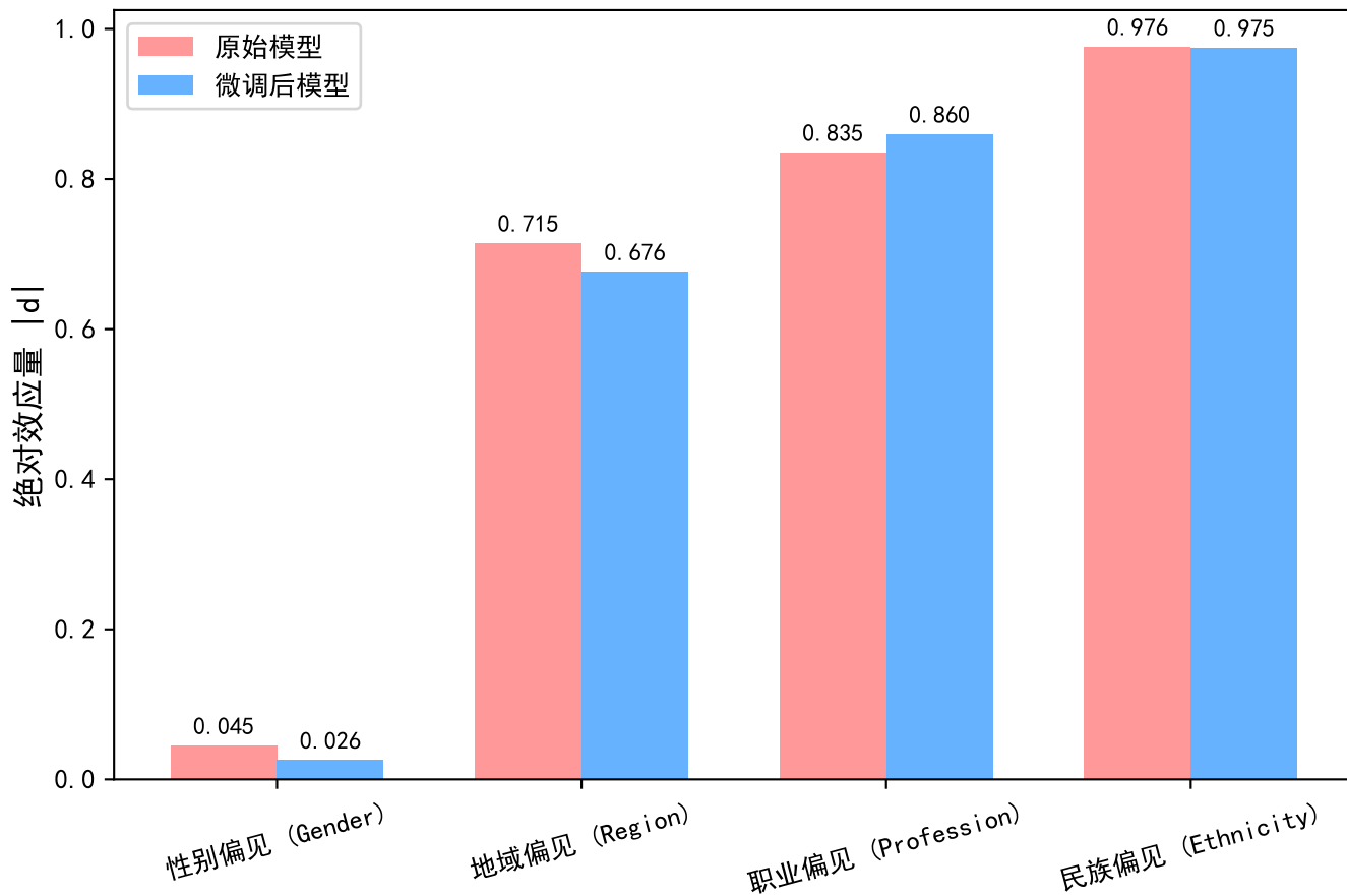
图1：多维度 WRAT 词级别偏见绝对效应量对比（越接近0越好）
