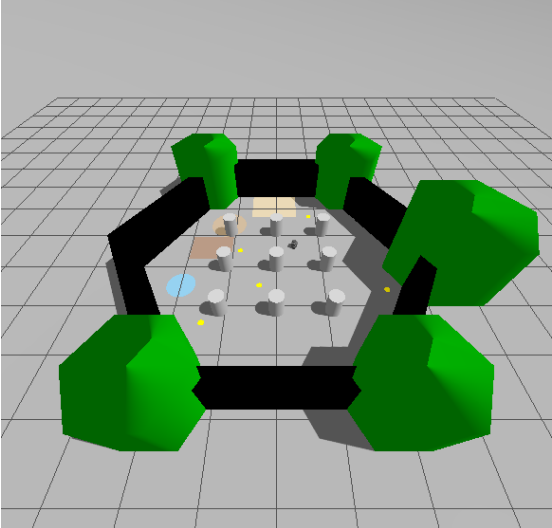
Окно Gazebo
