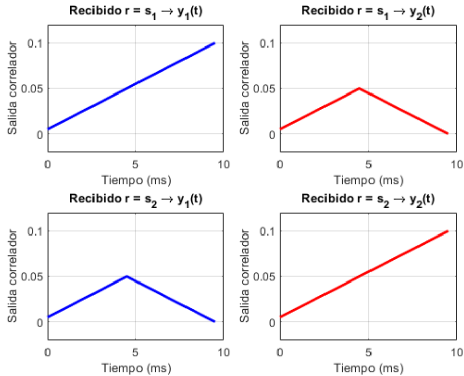
Ilustración 3: Símbolos demodulados por correlación
