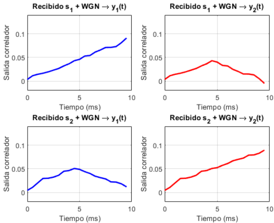
Ilustración 4: Salidas del banco de correladores bajo canal AWGN
