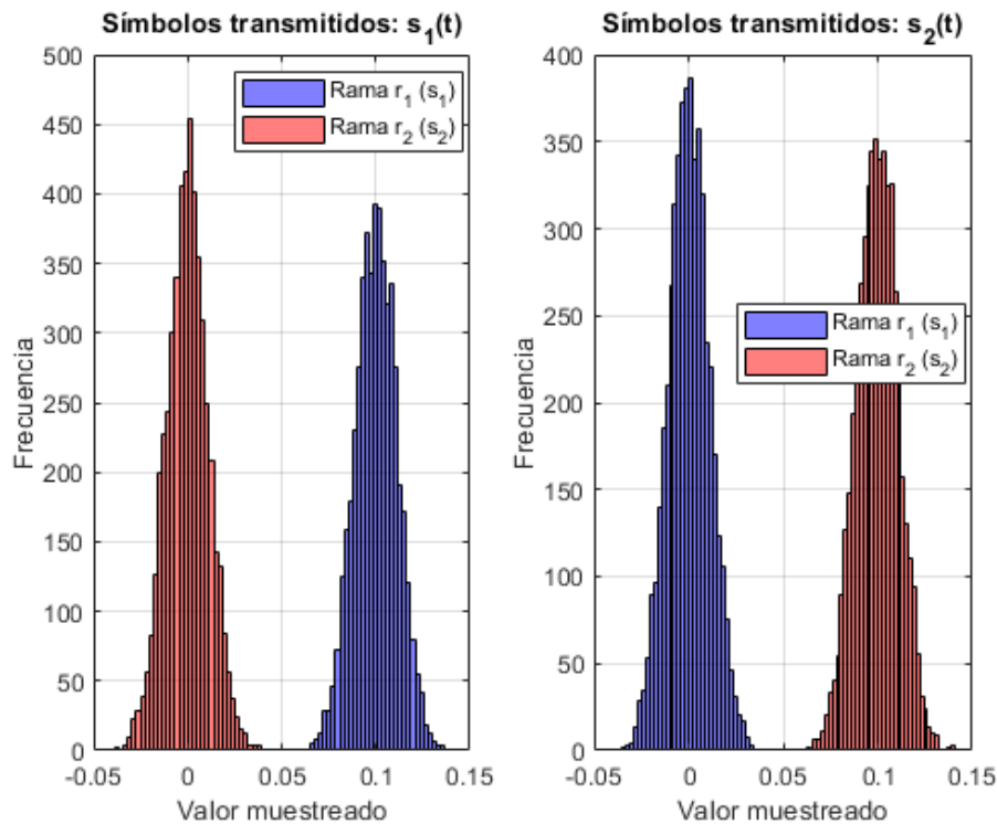
Ilustración 6: Histogramas de las salidas muestreadas en función de la transmisión de s_1(t) y s_2(t)
