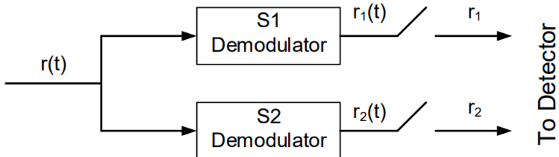
Ilustración 5: Esquema del demodulador de dos ramas usado
