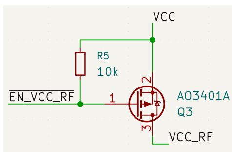
Rysunek 4.7: Tranzystor załączający linię zasilania nadajnika radiowego
