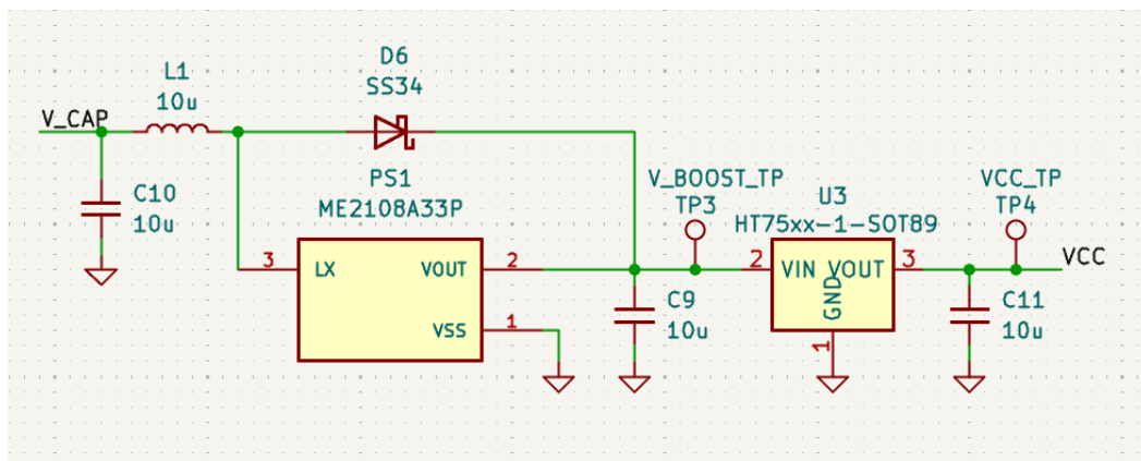
Rysunek 3.4: Układ regulacji napięcia oparty o przetwornicę step-up i regulator liniowy.
