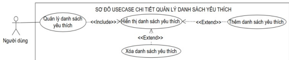
Hình 2.1: Sơ đồ use case quản lý danh sách yêu thích
