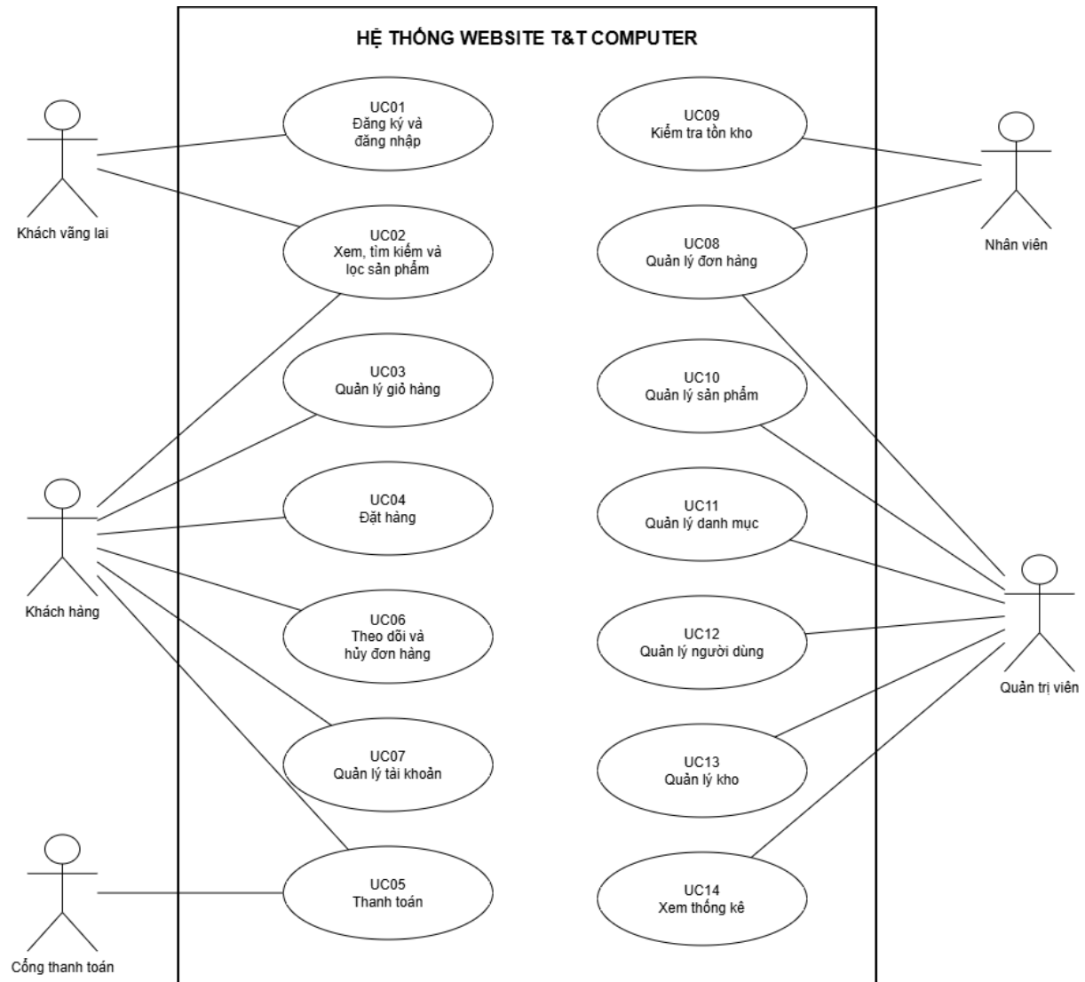
Hình 1: Biểu đồ Use Case tổng quát
